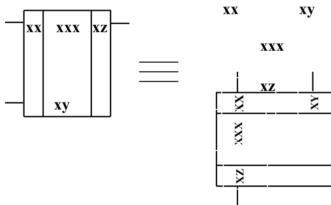
Рисунок 15 - УГО элементов цифровой техники (при повороте изображения)
