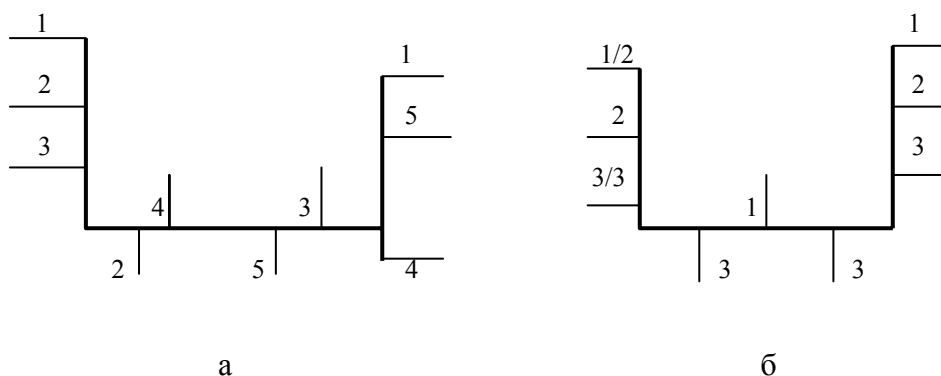
Рисунок 1 – Графическое слияние линий связи - линии групповой связи допускается выполнять утолщенными;
