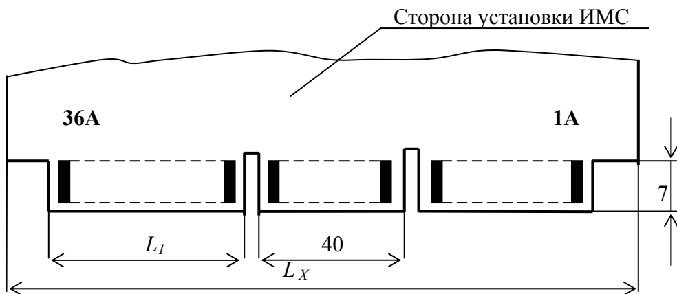
Рисунок 24 – Формирование контура платы и прорановка размеров
