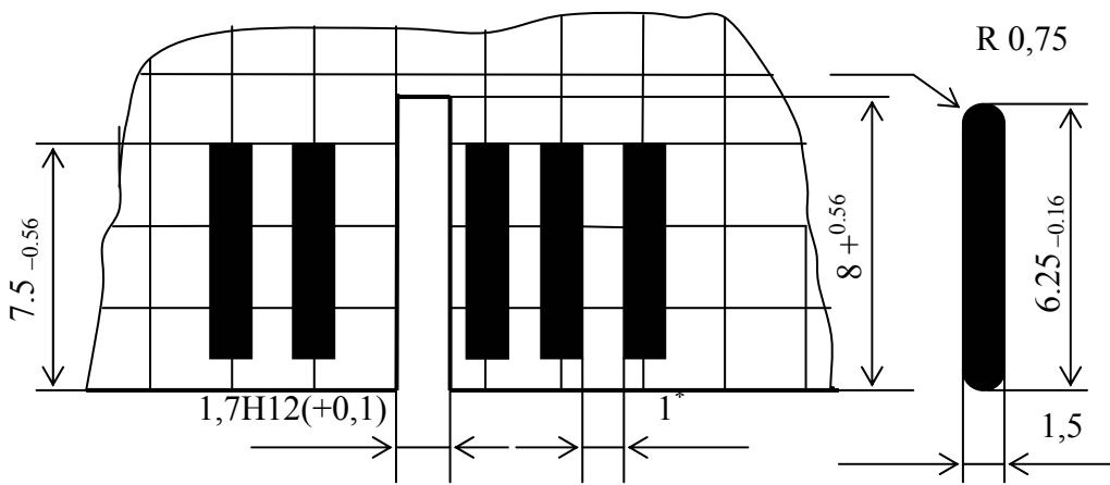
Рисунок 23 – Размеры и форма конечных печатных контактов (типа СНП) (1* - размер для справок)
