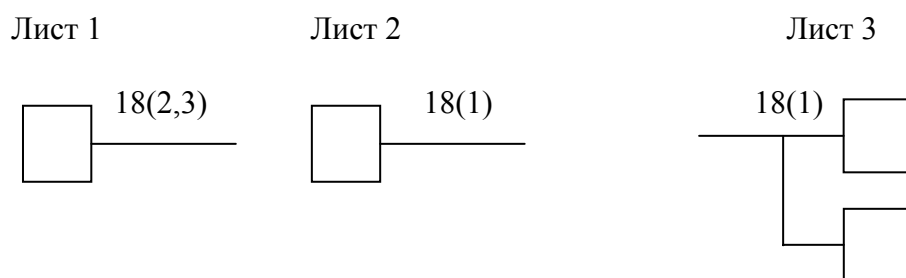
Рисунок 8 – Обозначение выходящих и входящих линий связи, имеющих продолжение на нескольких листах схемы
