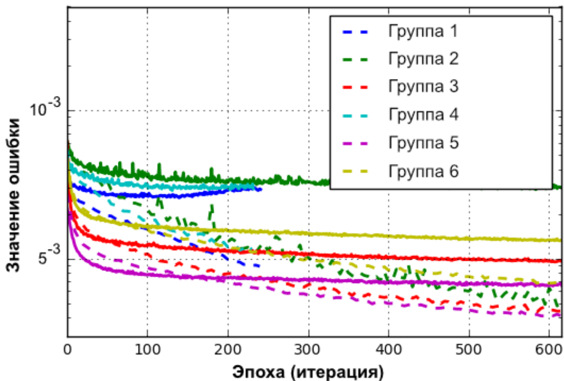
Рисунок 3.12 – График изменения значений ошибок в процессе обучения
