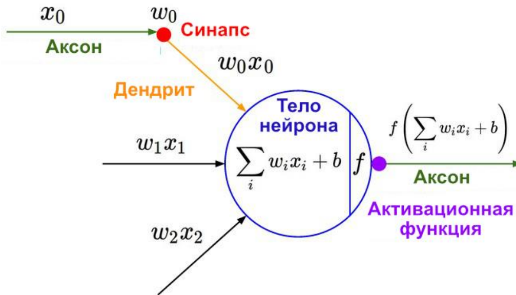
Рисунок 3.1 – Модель прохождения сигнала через нейрон
