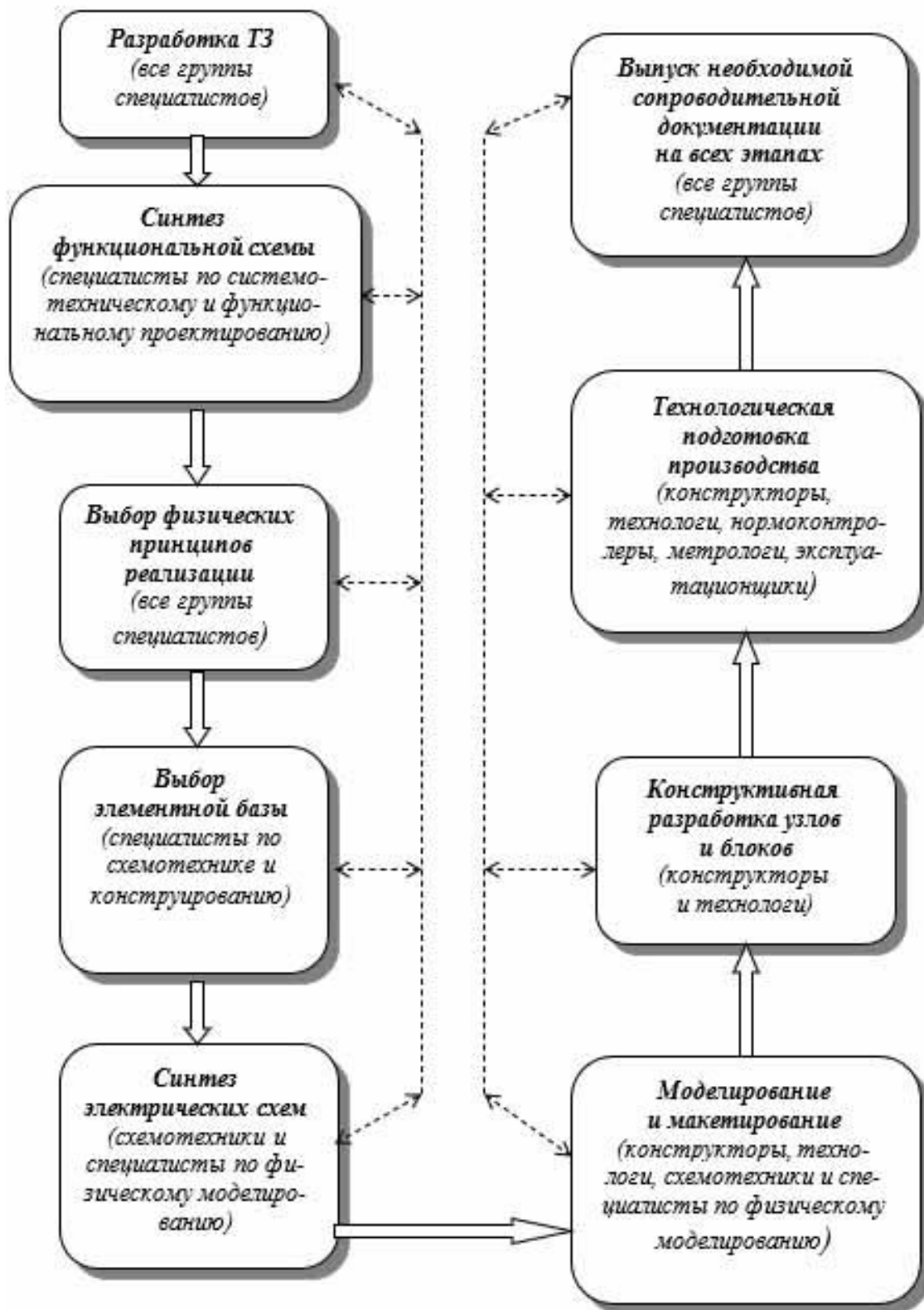
Рисунок 2.4 – Основные этапы проектирования технических систем
