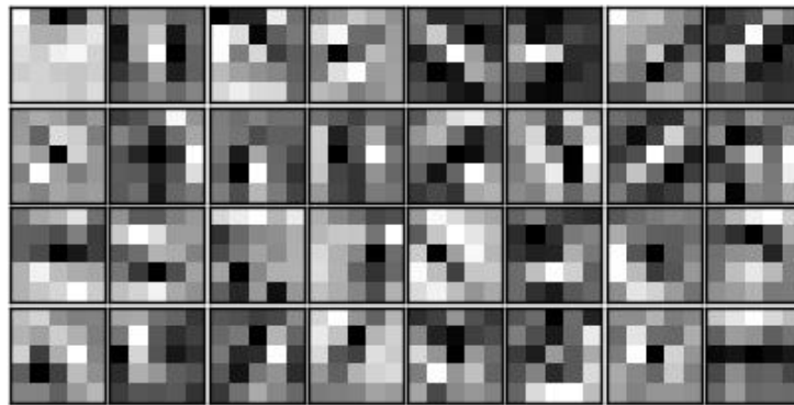
Рисунок 3.1 – Исходная визуализация
