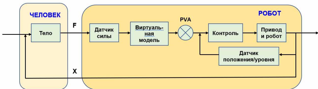
Рисунок 1.4 – Схема управления алгоритмом управления робота
