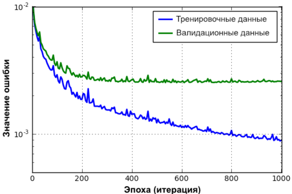
Рисунок 3.5 – График изменения значения ошибки в процессе обучения
