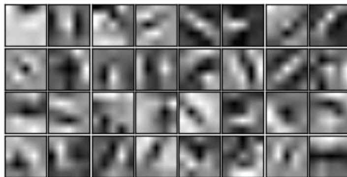
Рисунок 3.2 – Интерполированная визуализация
