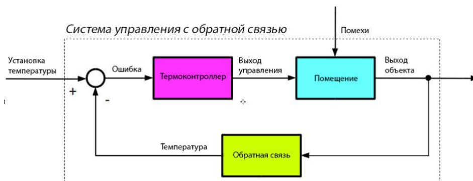
Рисунок 1.3 – Система управления с обратной связью
