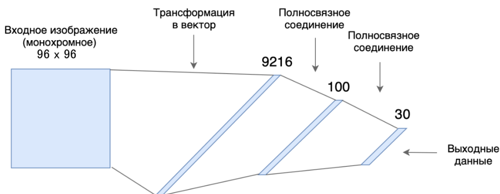
Рисунок 3.4 – Архитектура модели на основе неглубокой сети с одним скрытым слоем
