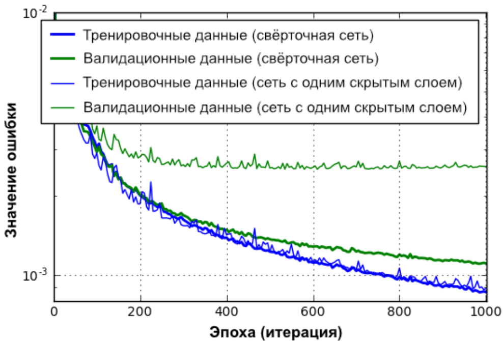
Рисунок 3.8 – График изменения значения ошибки в процессе обучения
