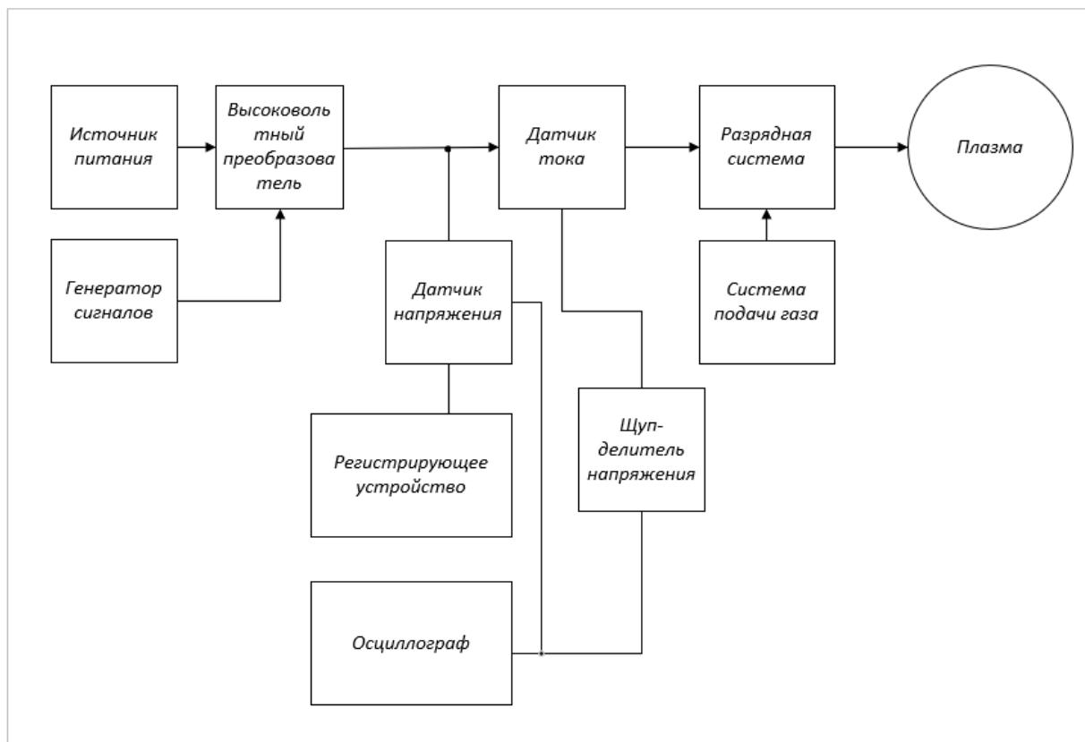
Рисунок 1 – Структурная схема лабораторного макета
