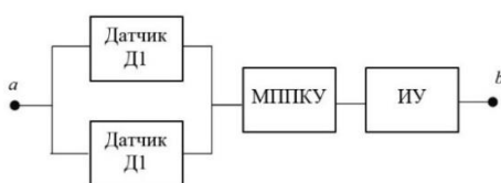
Рисунок 2 – Структурная схема надёжности исследуемой ЭСБ
