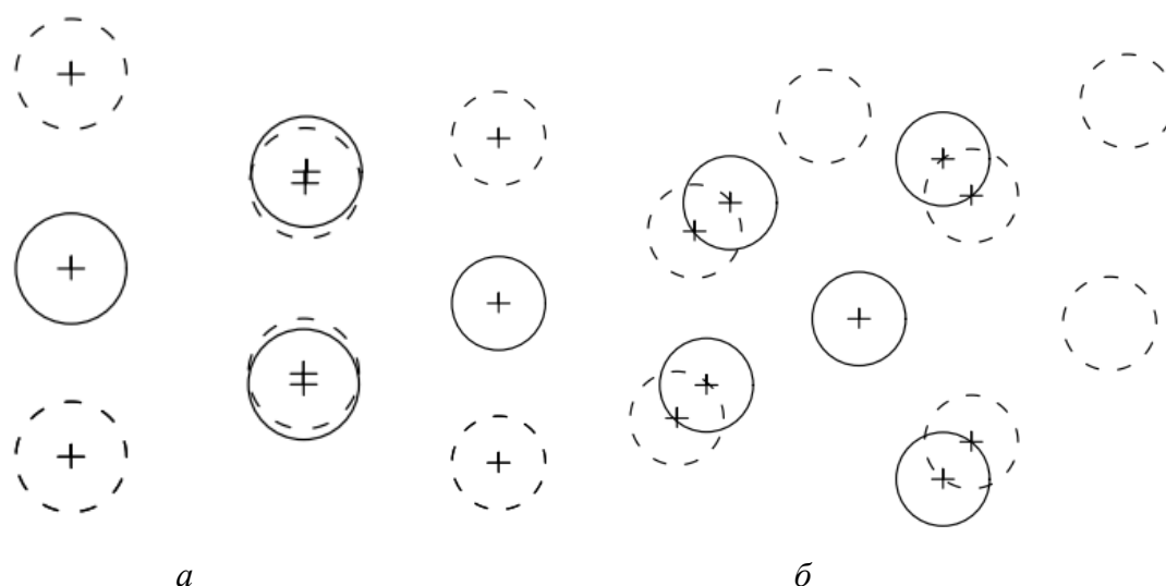
Рис. 3. Проекция базисной плоскости WSi_2 на плоскость кремния: a - \langle 111 \rangle ; b - \langle 100 \rangle . Сплошные окружности – атомы Si в WSi_2 , штриховые – в подложке
