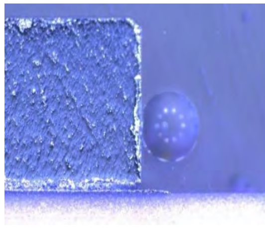
Рисунок 3 – Внешний вид изделий (вертикальный шлиф) загерметизированных с использованием окон с металлизацией на торце (а) и без металлизации (б)
