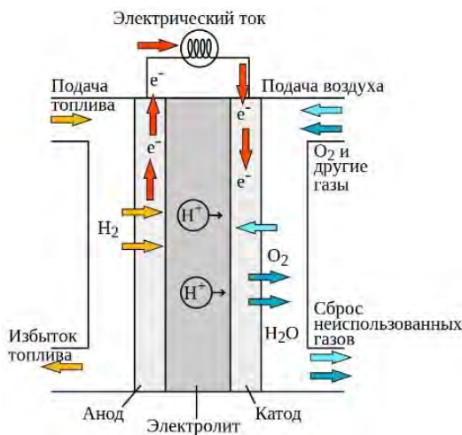
Рисунок 1 – Водородно-кислородный топливный элемент
