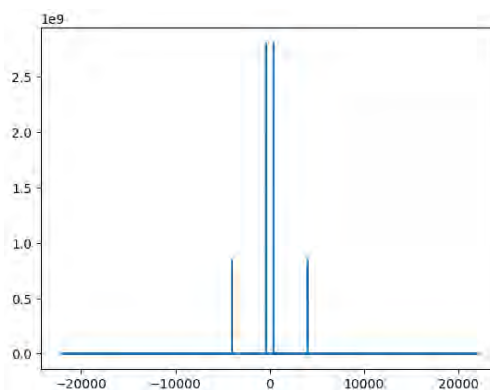
Рисунок 2 – Результат FFT-преобразования
