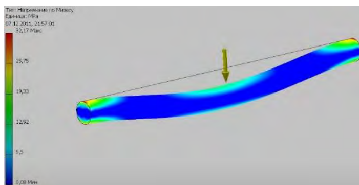
Рисунок 2 – Расчет на прочность детали
