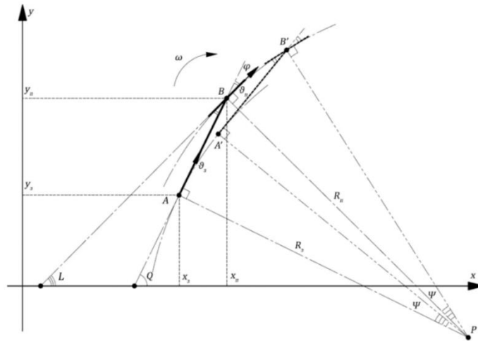
Рисунок 1 – Кинематическая схема движения платформы
