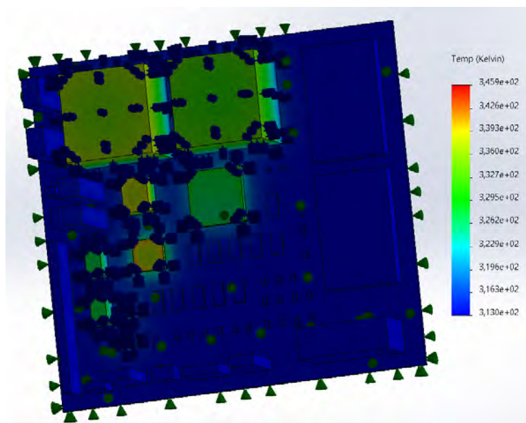
Рисунок 3 – Результат моделирования тепловых процессов
