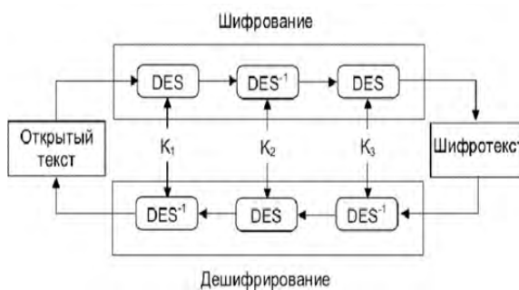
Рисунок 4 – Схема работы DES
