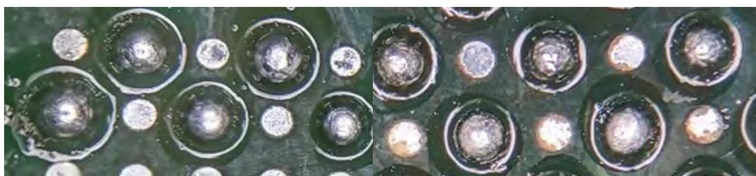
Рисунок 2 – Внешний вид шариков, образованных из паяльной пасты
