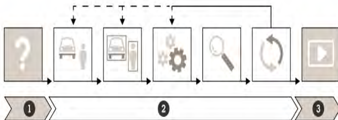
Рисунок 1 – Машинное обучение
