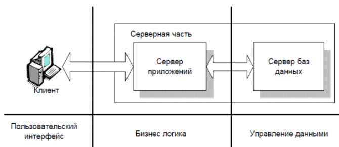
Рисунок 1 – Архитектура веб-сайта
