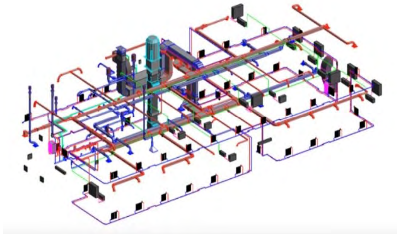
Рисунок 1 – 3d схема рабочей вентиляции со встроенными сплит-системами
