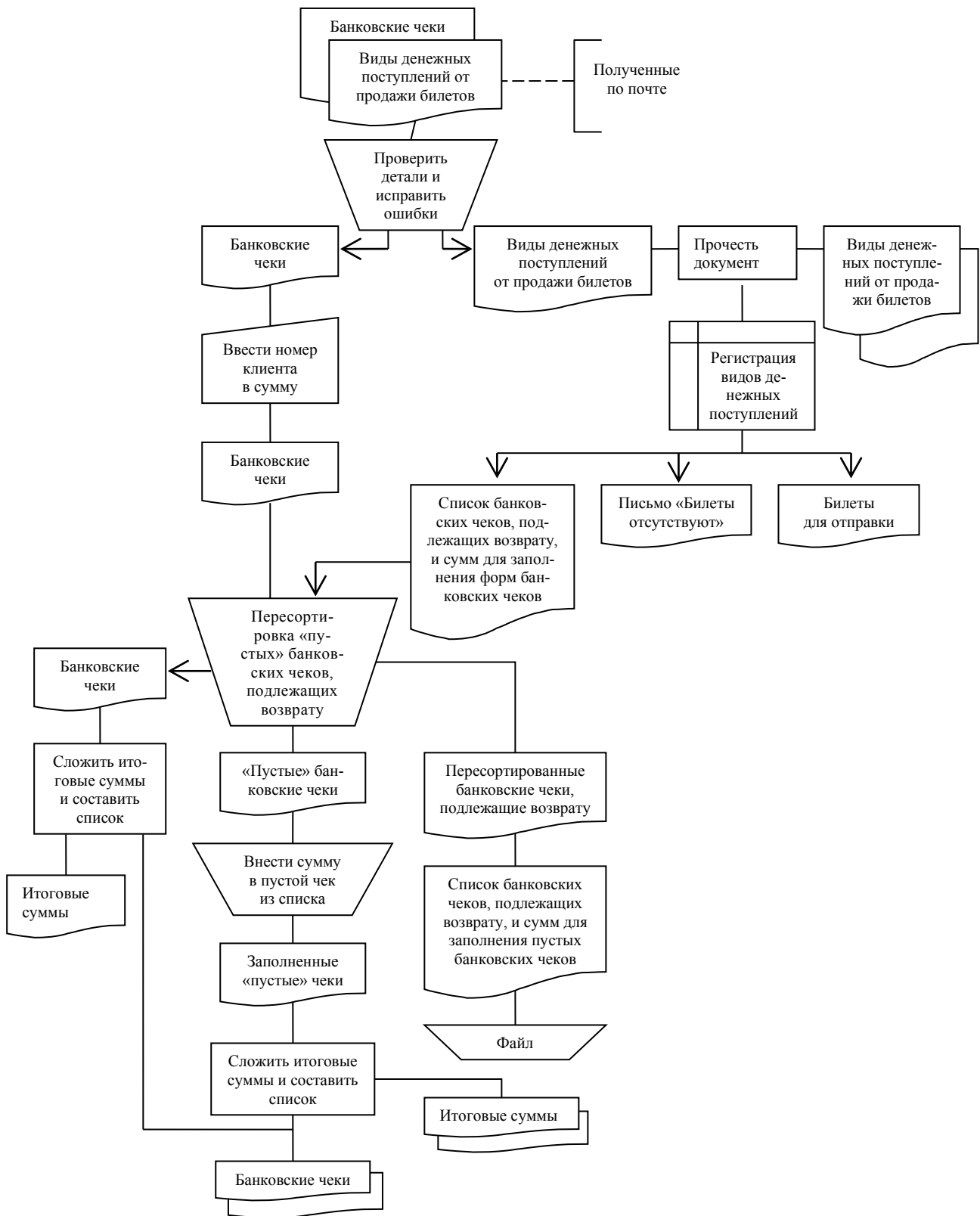
Рисунок 3.27 – Схема данных
