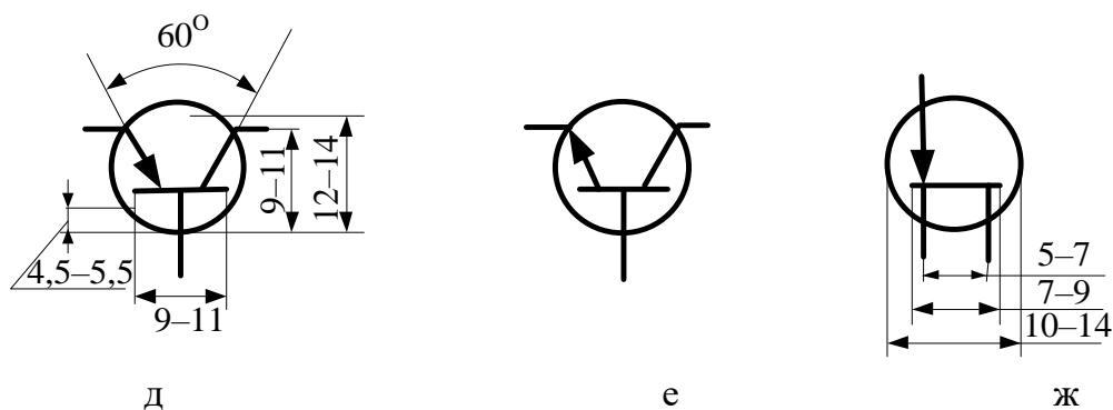
Рисунок 3.10 – Условные графические обозначения полупроводниковых приборов (к пункту 3.3.7)
