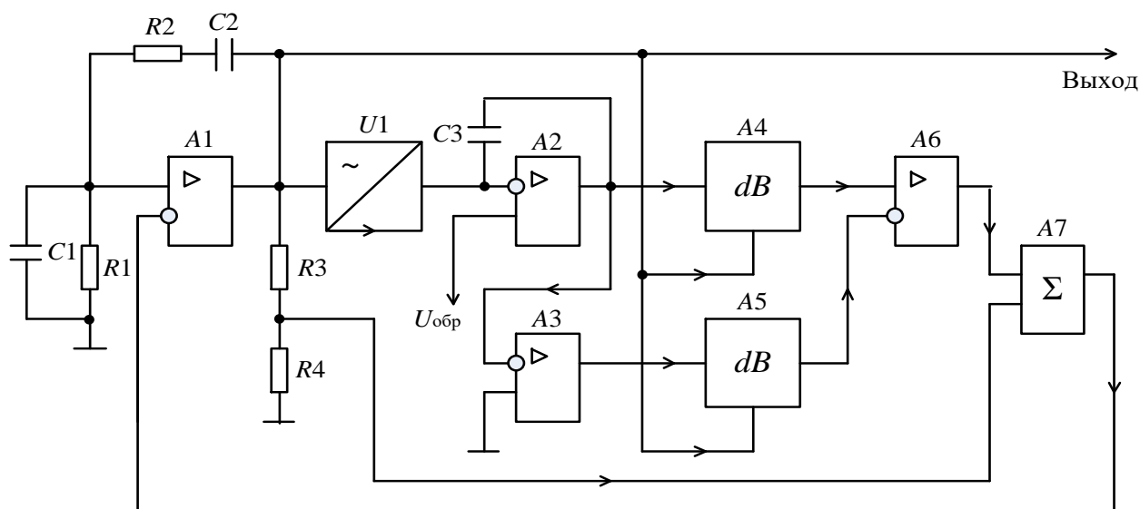
Рисунок 3.20 – Схема электрическая функциональная технического устройства
