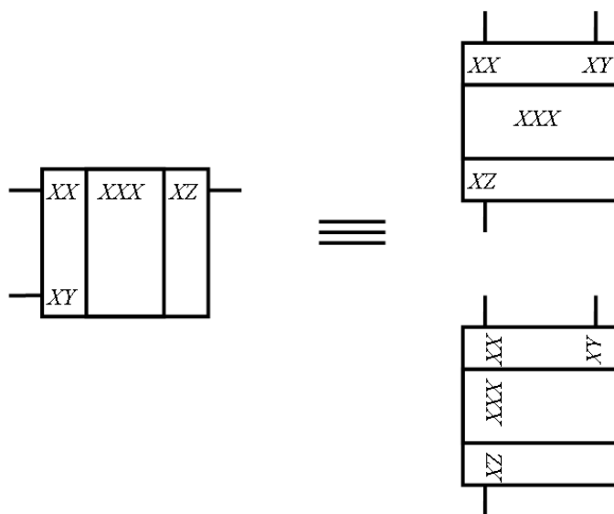
Рисунок 3.14 – Расположение выводов элементов цифровой техники (к пункту 3.4.4)
