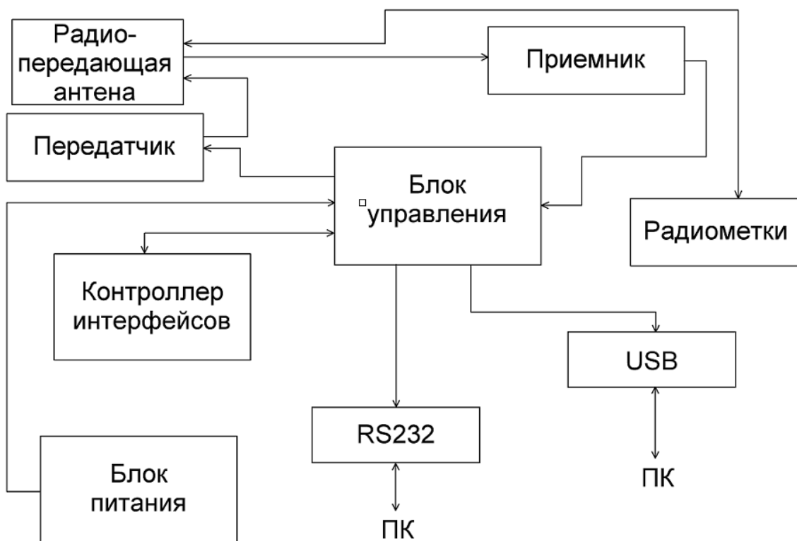
Рисунок 1 – Схема электрическая структурная разработанной системы
