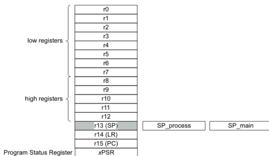
Рисунок 1 – Регистры arm-m3/m4-процессора
