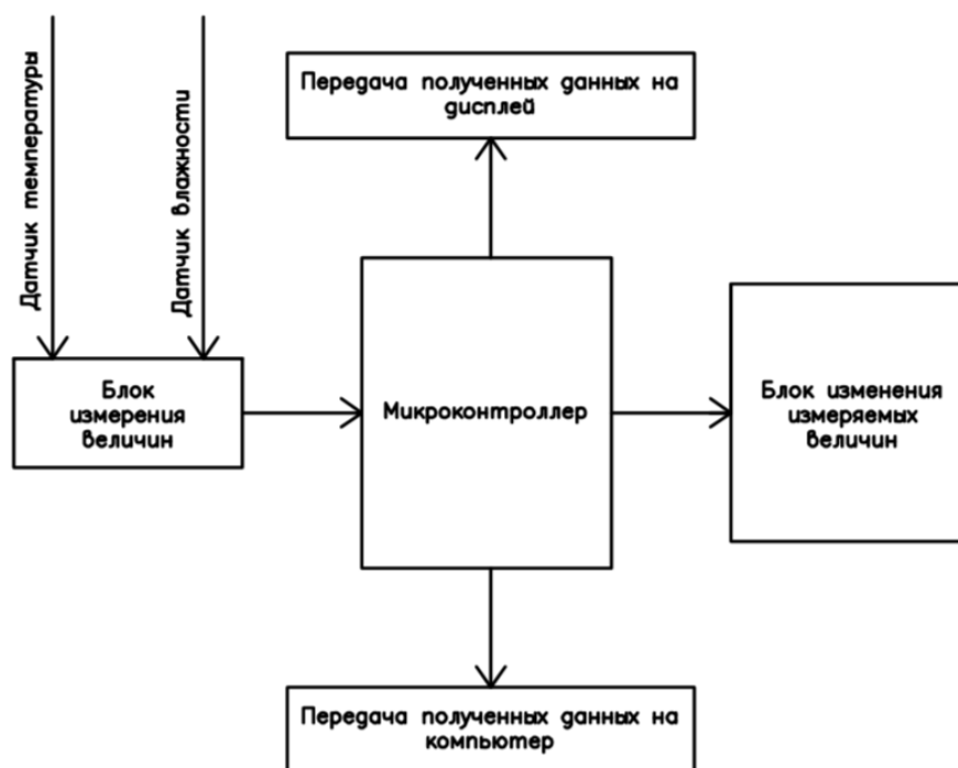
Рисунок 1 - Структурная схема системы контроля параметров картофелехранилища
